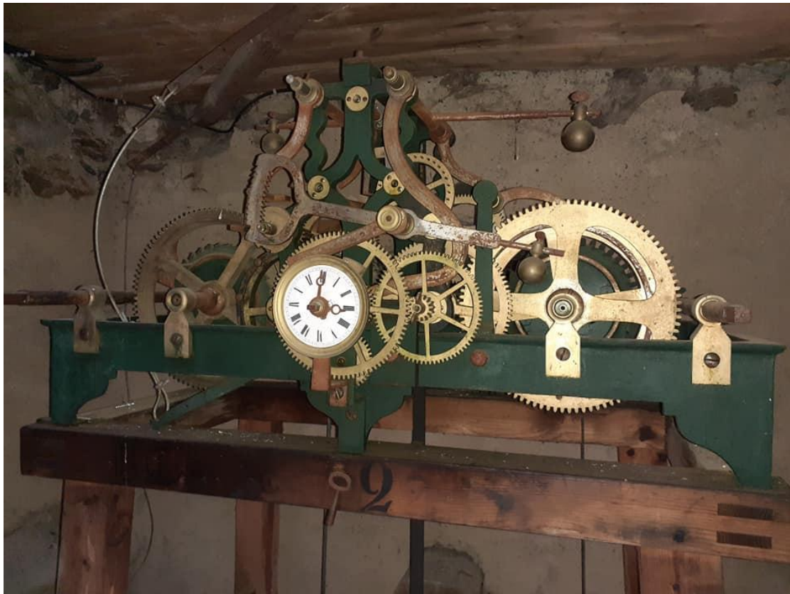
Mécanisme de l'ancienne horloge de l'église
